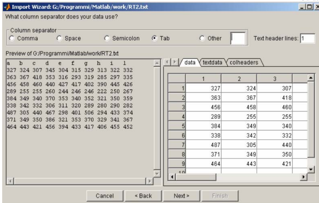
Figura 11. L'Import Wizard.
